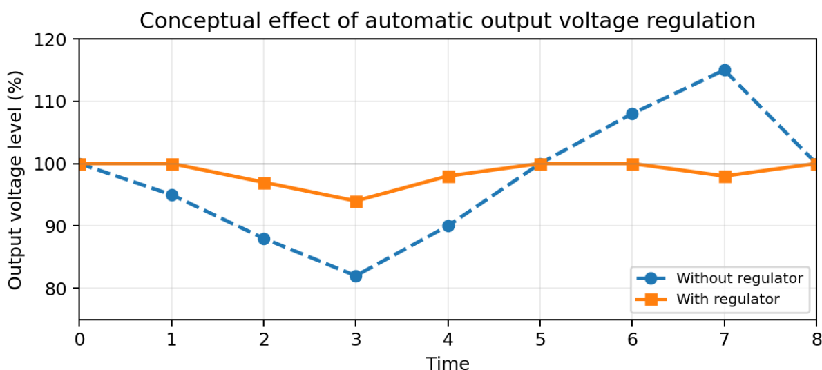
نمودار ۱- اثر فاندکشن AVR بر روی پایداری ولتاژ خروجی درایو
