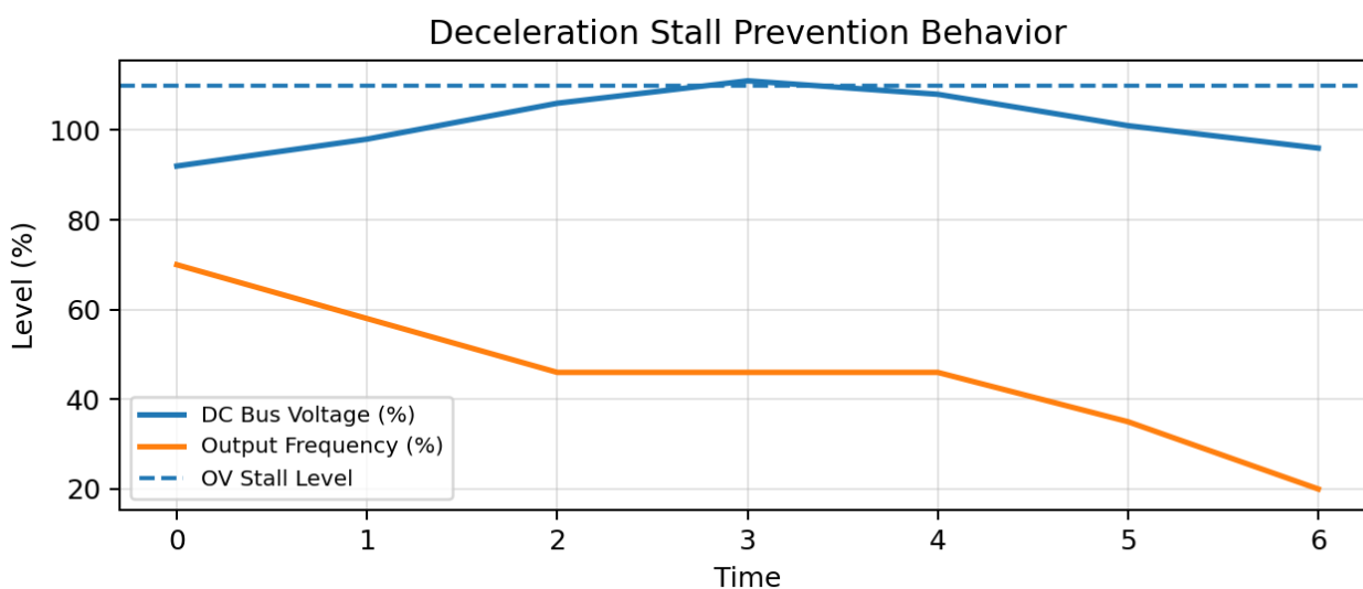
نمودار (۲): رفتار مفهومی جلوگیری از اضافه‌ولتاژ در زمان کاهش سرعت
