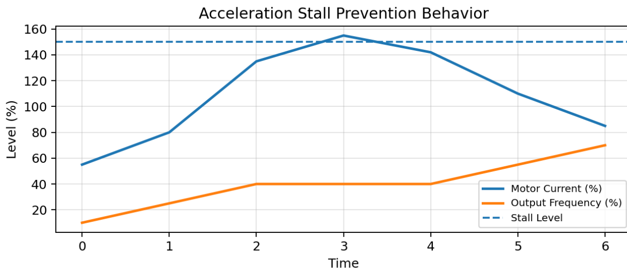
نمودار (۱): رفتار مفهومی جلوگیری از استال در زمان شتاب‌گیری
