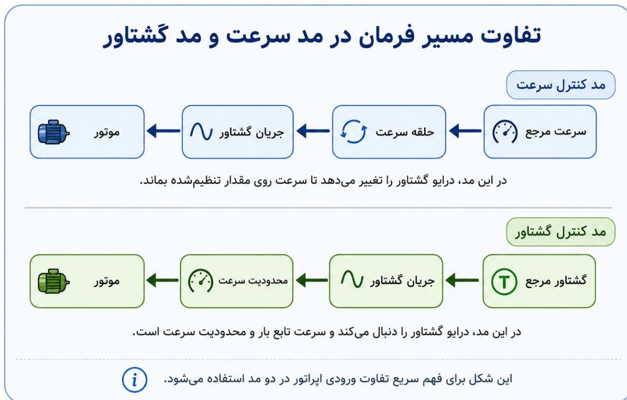
شکل (۱): مقایسه مسیر فرمان در مد سرعت و مد گشتاور
