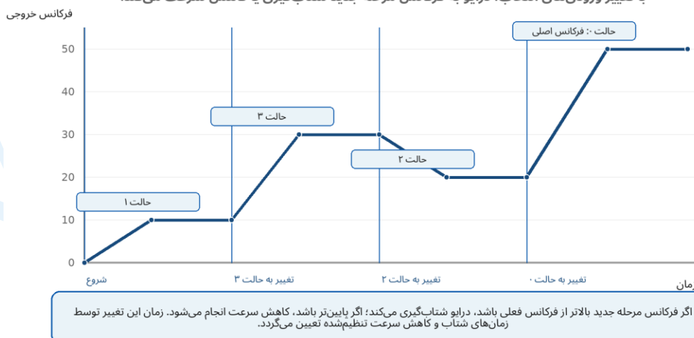
شکل (۲): نمونه تغییر فرکانس خروجی هنگام تغییر حالت چندمرحله‌ای
